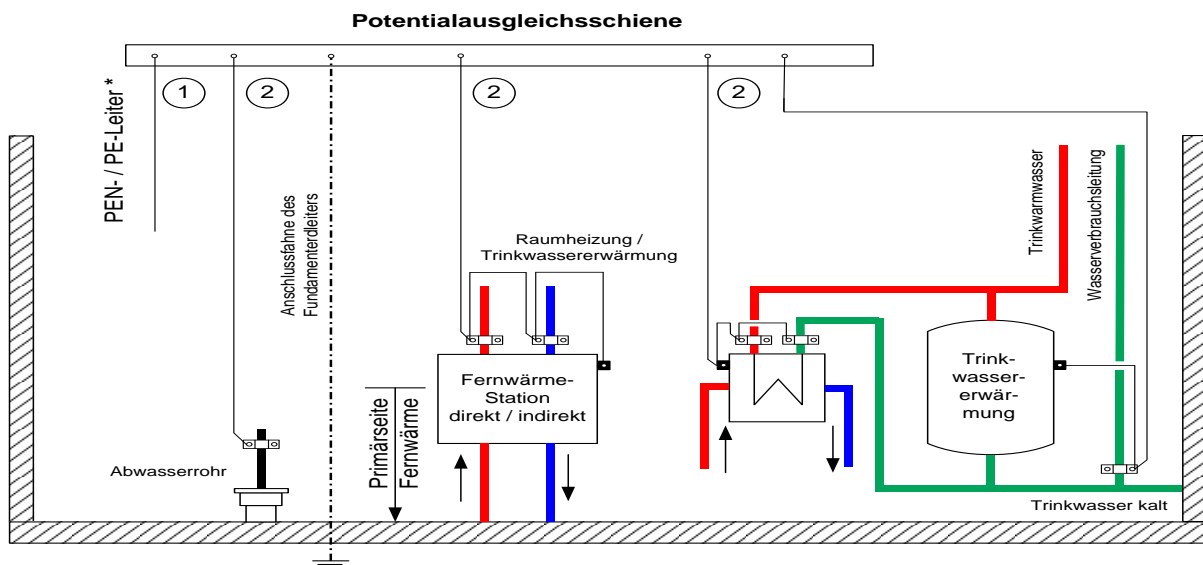
Abbildung 2: Beispiel eines Potentialausgleichs
