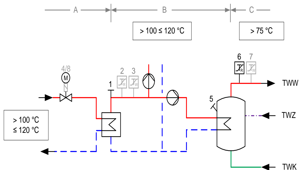
Abbildung zur Tabelle 9: Erforderliche sicherheitstechnische Ausrüstung nach Zeile 5; grau dargestellte Komponenten nicht erforderlich
