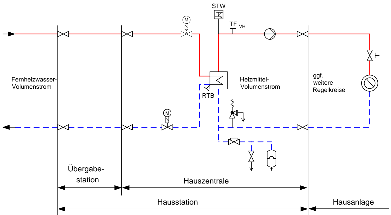
Abbildung 8: Hauszentrale-Raumheizung Prinzipschaltbild für den indirekten Anschluss
