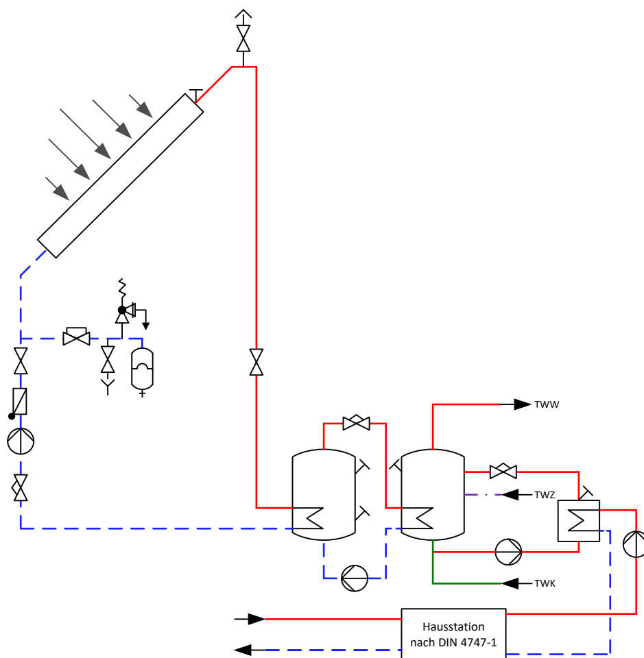
Abbildung 13: Solaranlage mit Pufferspeicher und Trinkwassererwärmer mit außen liegendem Wärmeübertrager für die Nachheizung
